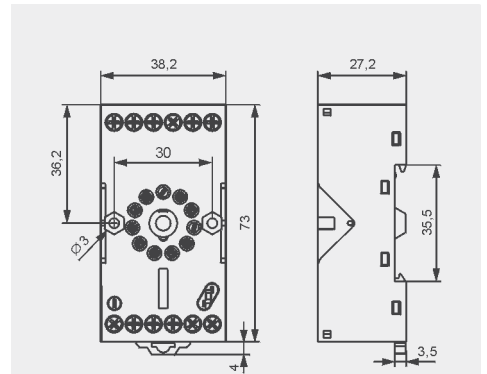
Module type 21, 41
